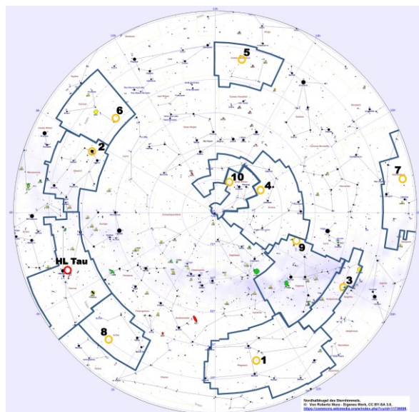
Sternkarte der nördlichen Himmelshalbkugel mit den 10 Stationen der Exoplaneten-tour. Zu jeder Station gibt es eine Stationskarte . Die Stationen liegen in 10 verschiedenen Sternbildern, die entsprechend der wissenschaftlichen Festlegung als begrenzte Gebiete an der scheinbaren Himmelshalbkugel markiert sind. Dies sind hier:
